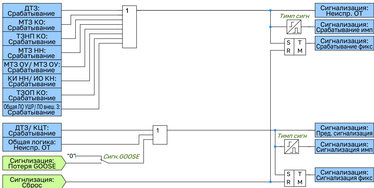
Рисунок 2.17 – Функциональная схема логики сигнализации
