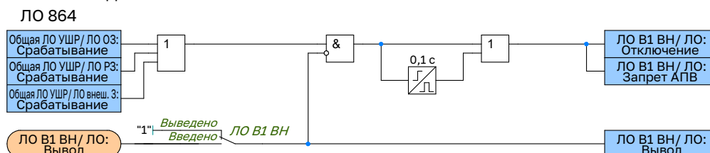
Рисунок 2.15 – Функциональная схема логики отключения В1 ВН
